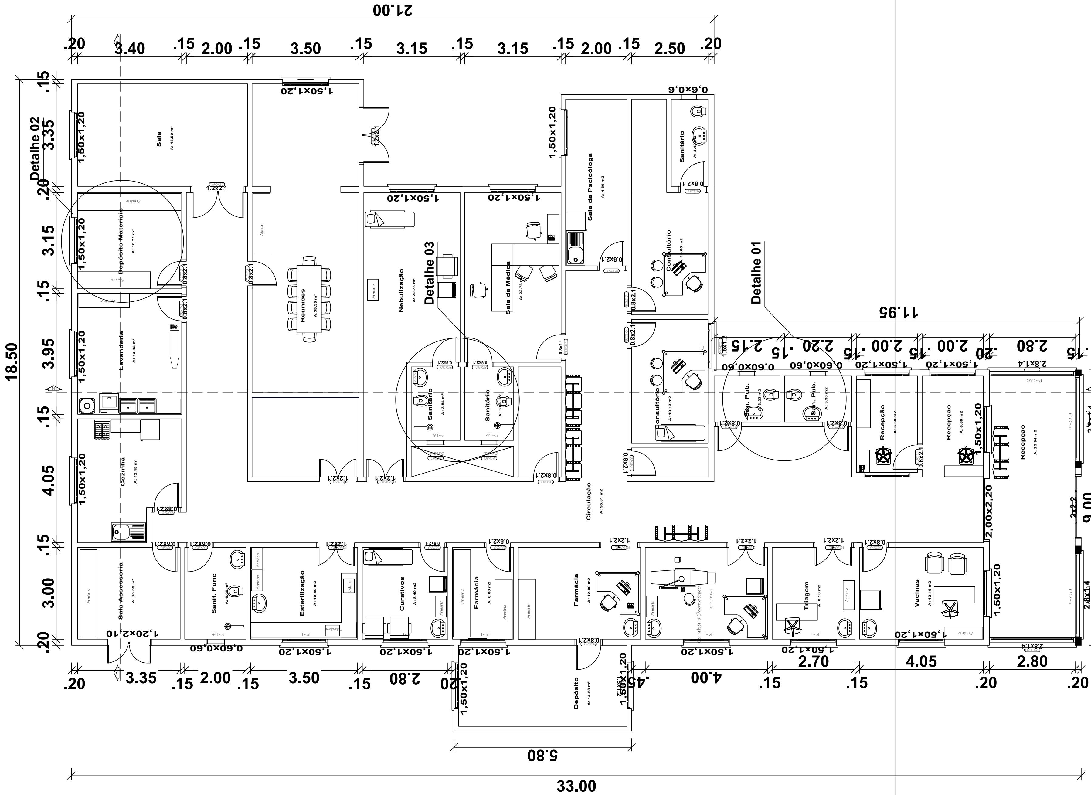
PLANTA BAIXA - UBS
