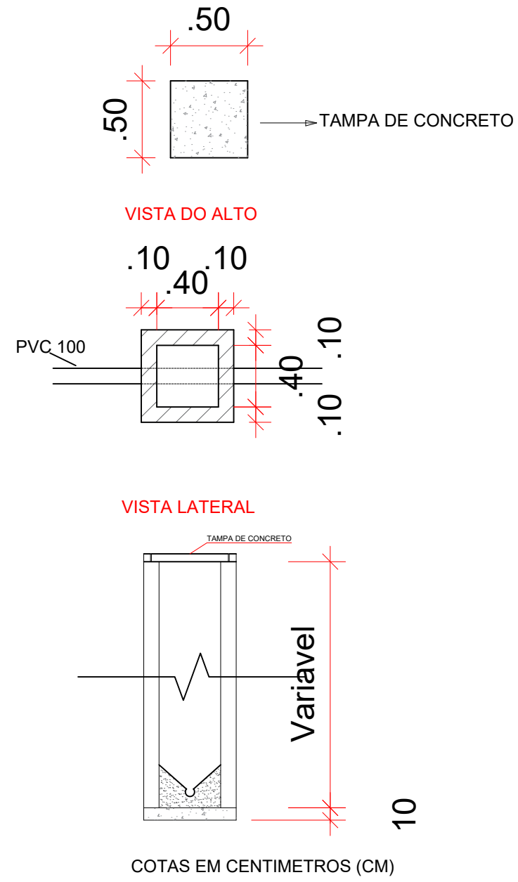
DETALHE DA CAIXA DE INSPEÇÃO - CI
